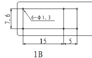
安装脚位图 (底视图) PCB Layout (Bottom view)
